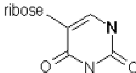
Pseudouridine
